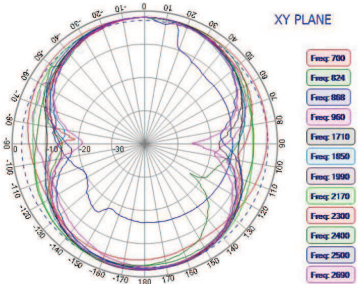
LTE Antenna
